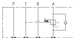
油圧記号
