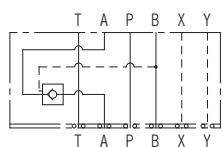
(Aポートパイロットチェック弁) 油圧記号
