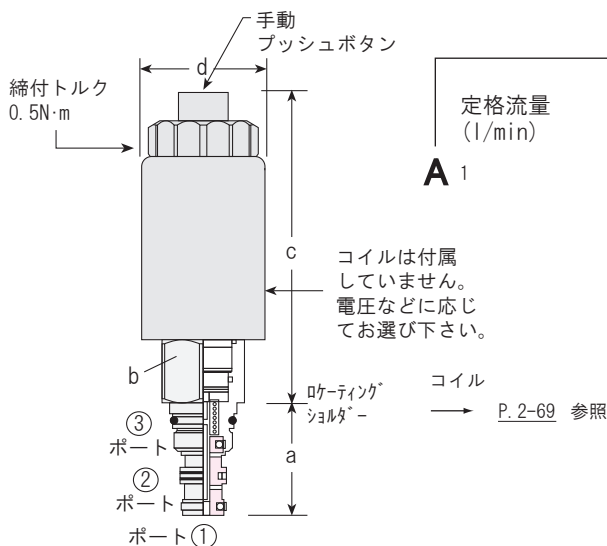
シリーズ P (DBAF-MCN)
