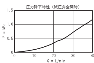
シリーズ 3 (PVHA-LAN)
