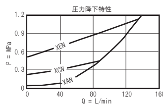
シリーズ 2 (CXFA-X**)
