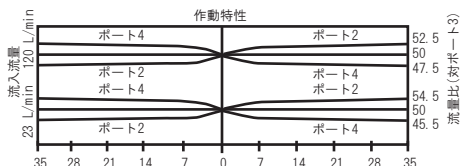
シリーズ 3 (FSES-XAN)
