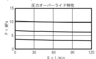
シリーズ 4 (PBJB-LAN)
