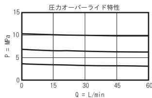
シリーズ 3 (PBHB-LAN)
