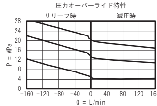
シリーズ 3 (PRHB-LAN)
