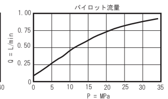
シリーズ 4 (RSJC-LAN)
