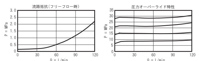
シリーズ 4 (CBIG-LJN)
