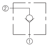
チェック弁（１）
