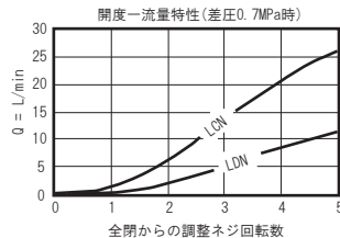
シリーズ 1 (NFCC-***)
