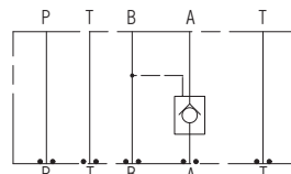
油圧記号
