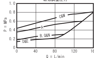
シリーズ 4 (RPKC-LAN)
