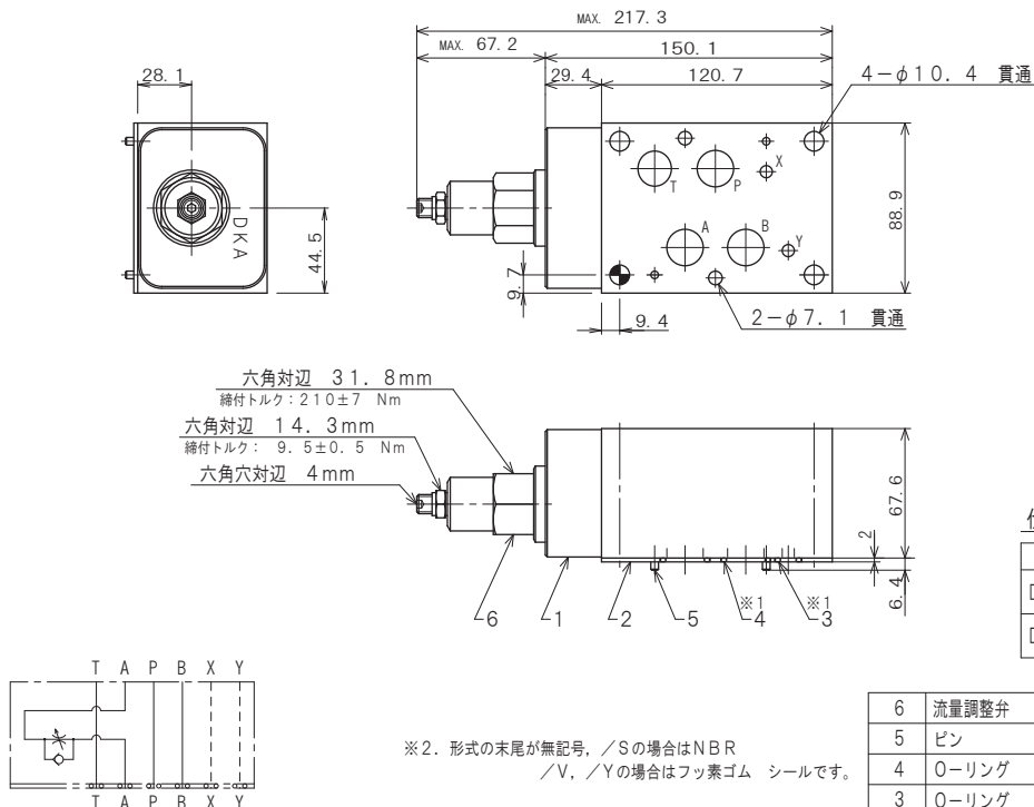
(Aポートメータアウト流量調整弁) 油圧記号
