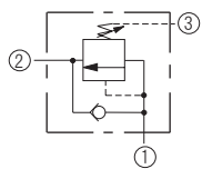
直動形シーケンス弁 (チェック弁付)
