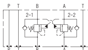
油圧記号
