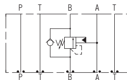
油圧記号
