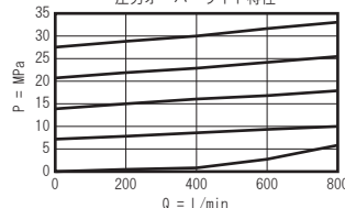
シリーズ 3 (RPIC-LAN)
