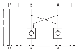
油圧記号
