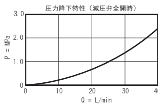
シリーズ 1 (PBDB-LAN)
