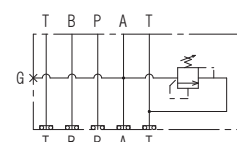
(A-Tリリーフ弁) 油 圧 記 号
