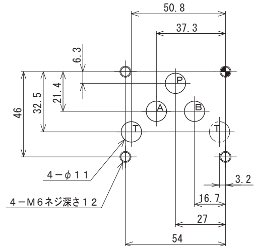
マニホールド加工寸法 (ISO 05 相当)
