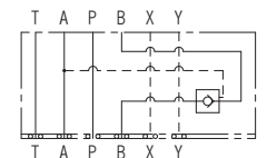
(Bポートパイロットチェック弁) 油 圧 記 号
