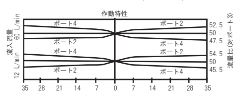
シリーズ 2 (FSDS-XAN)
