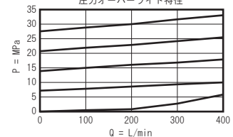
シリーズ 4 (RPKC-LAN)
