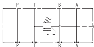
油圧記号
