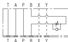
(Bポートメータアウト流量調整弁) 油 圧 記 号
