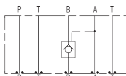
油圧記号
