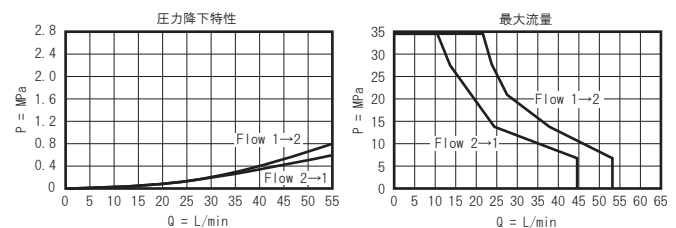
シリーズ 1 (DLDF-MHN)
