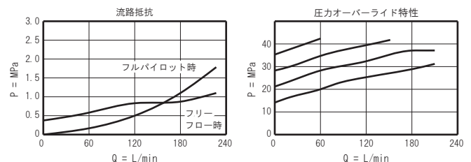
シリーズ 3 (MWGG-LJN)
