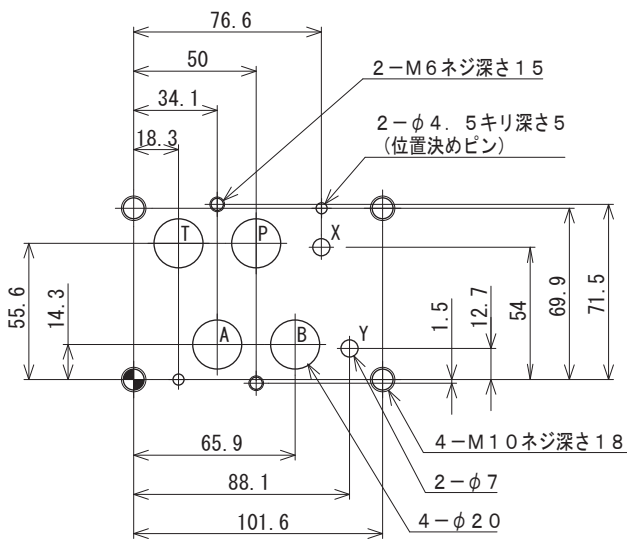
マニホールド加工寸法 (ISO 07 相当)
