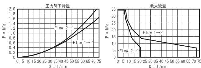
シリーズ 1 (DTDF-MCN)
