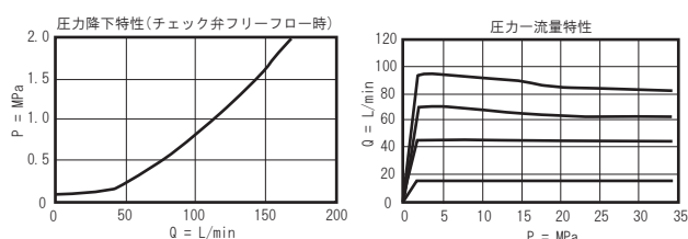
シリーズ 3 (FDEA-LAN)
