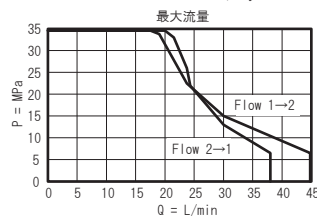
シリーズ 1 (DMDF-MNN)
