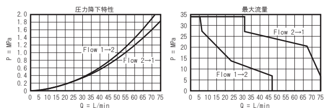
シリーズ 1 (DTDF-MHN)
