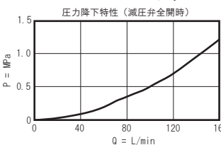
シリーズ 3 (PBHB-LAN)
