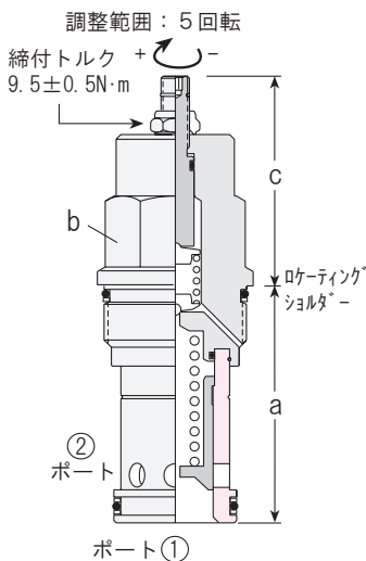
シリーズ 0 (RPCC-LAN)
