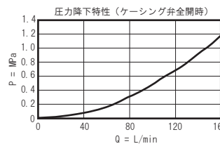
シリーズ 2 (RSFC-LAN)
