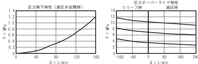
シリーズ 3 (PVHB-LAN)
