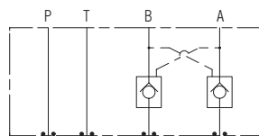
油圧記号
