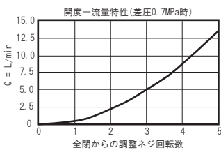
シリーズ 4 (NFFC-***)
