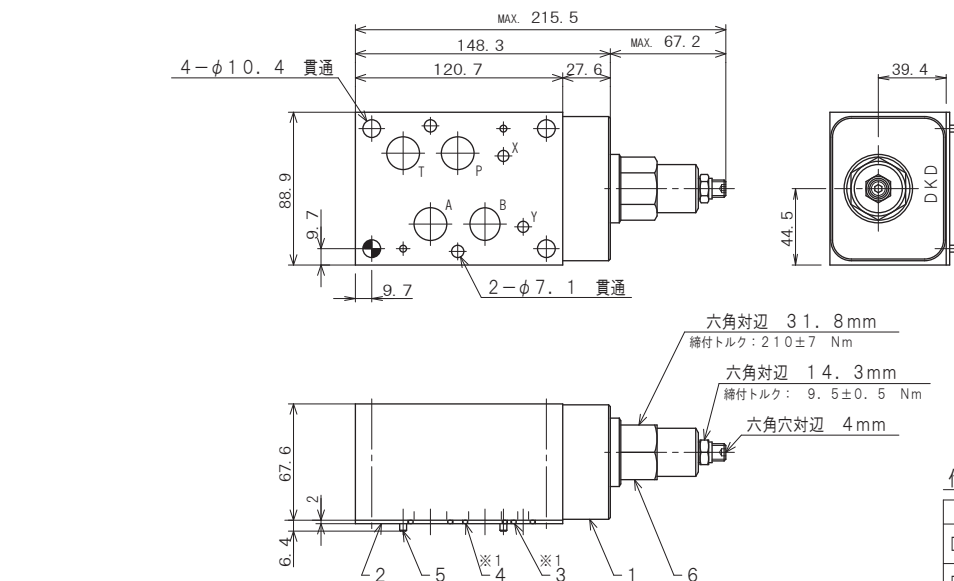
(Bポートメータイン流量調整弁) 油圧記号
