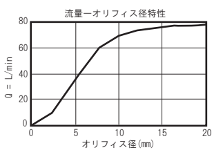
シリーズ 1 (LPDC-XHN)
