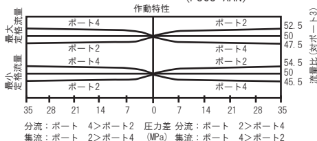
シリーズ 1 (FSBS-XAN) (FSCS-XAN)
