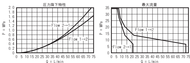
シリーズ 1 (DTDF-MCN)
