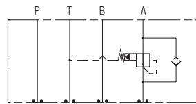
油圧記号
