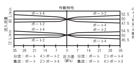
シリーズ 2 (FSDS-XAN)
