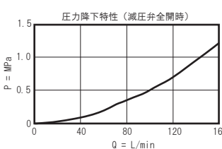
シリーズ 3 (PPHB-LAN)
