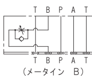
(メータイン B)
