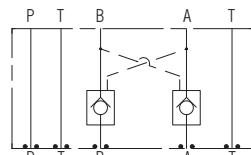
油圧記号
