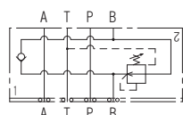
油圧記号
