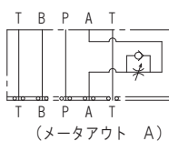
(メータアウト A)
