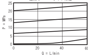
シリーズ 1 (RPEC-LAN)
