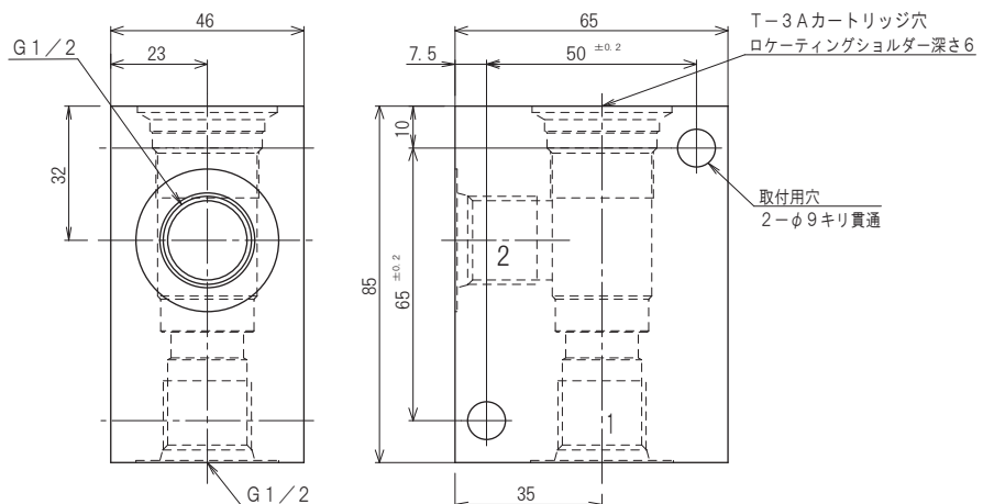
アングルタイプ
