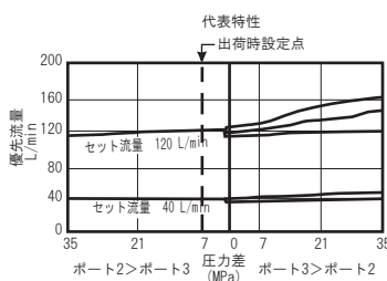
シリーズ 4 (FRFA-XAN)
