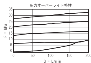
シリーズ 3 (RVGD-LAN)
