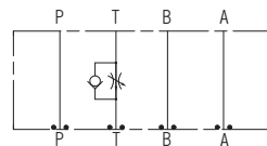
油圧記号
