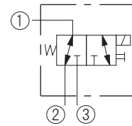
ノーマルオープン ① - ②
