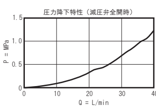
シリーズ 3 (PPHB-LAN)
