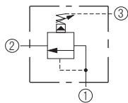
バランス形シーケンス弁
