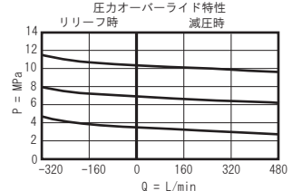
シリーズ 4 (PPJB-LAN)
