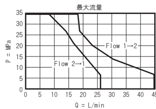
シリーズ 1 (DMDA-MNN)
