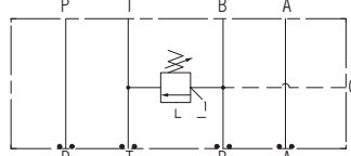
油圧記号
