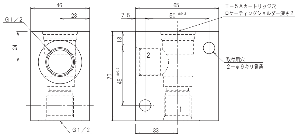
アングルタイプ
