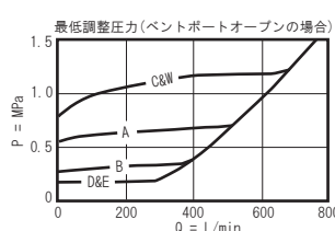
シリーズ 4 (RVID-LAN)
