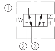
ノーマルオープン ① - ③
