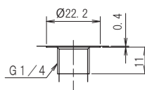
ゲージポート形状
