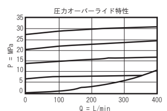
シリーズ 4 (RVID-LAN)
