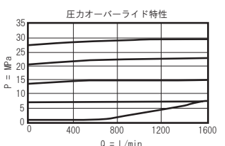
シリーズ 4 (RVID-LAN)
