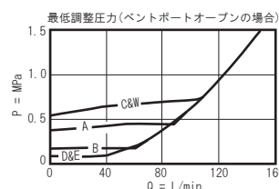
シリーズ 2 (RVED-LAN)
