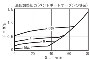
シリーズ 1 (RVCD-LAN)
