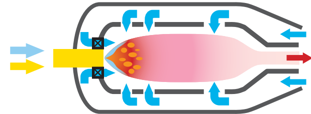
蒸汽 / 喷水方式图
