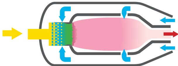
稀薄预混燃烧方式图
