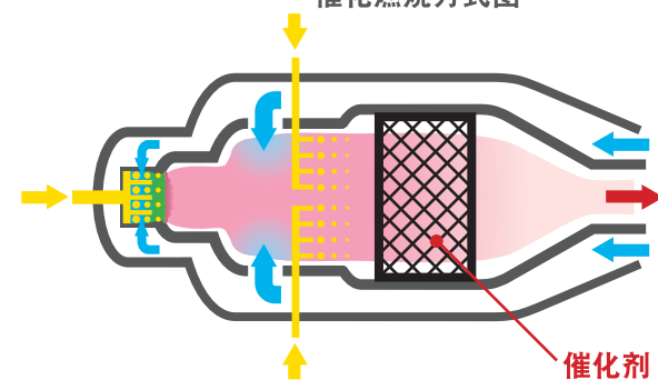
催化燃烧方式图
