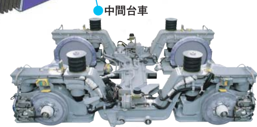
●中間台車
