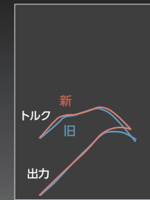
新 旧 トルク 出力 エンジン回転数 出力特性
