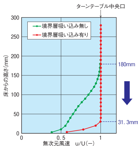
図2 境界層吸い込み装置の有無による境界層特性 Fig. 2 Effect of boundary layer absorber on boundary layer properties
