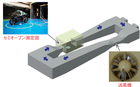
図1 風洞概要
