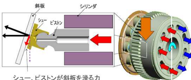
斜板形モータの作動原理
